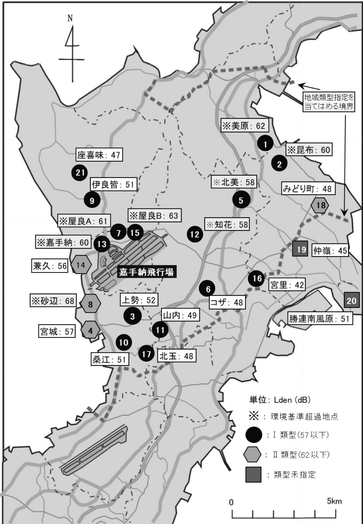
図7-2-1 嘉手納飛行場周辺における航空機騒音測定結果（平成30年度）
