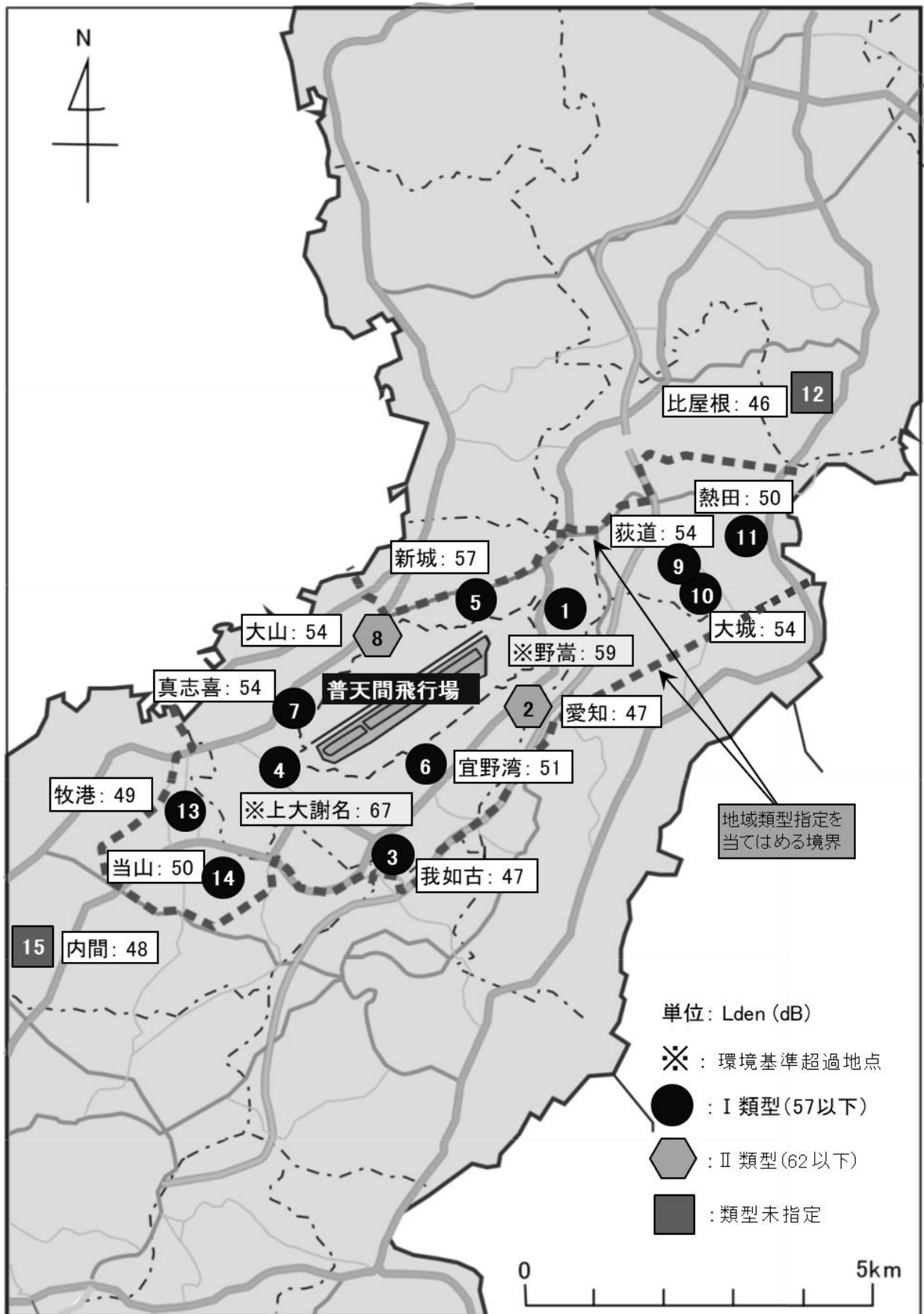
図7-2-2 普天間飛行場周辺における航空機騒音測定結果（平成30年度）
