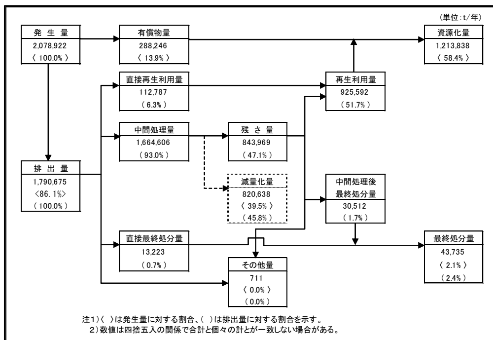
図8-2-4 産業廃棄物処理・処分フロー（平成28年度）
