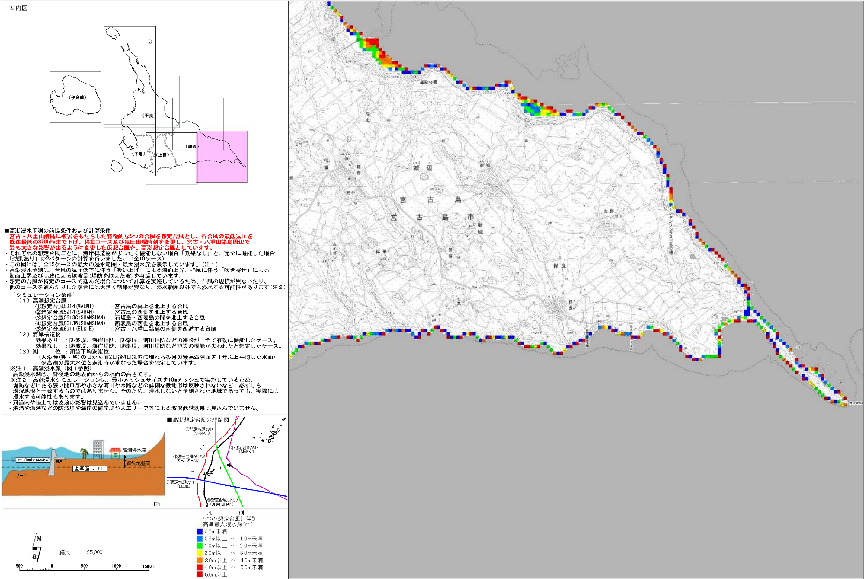
高潮浸水予測図 市町村別 宮古島市(4／8)
