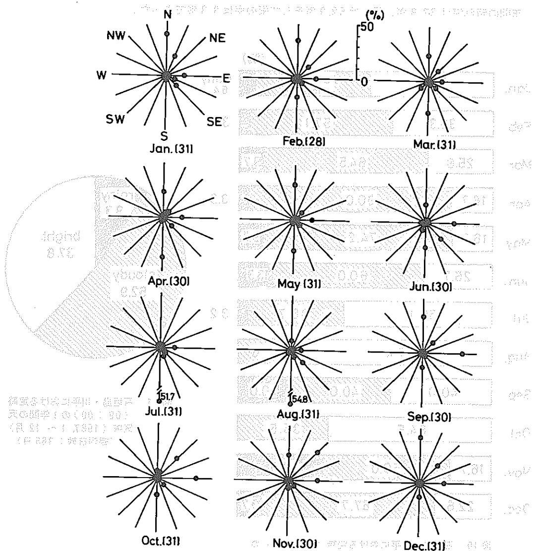
図12 石垣島・川平における定時(09:00)の月別風向率(1987.1~12月) ( ) : 観測日数
