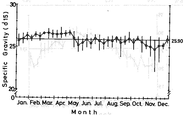
図9. 川平湾表層比重 ( \sigma_{15} ) (1987.1～12月) 旬別平均及び旬中最高最低比重 (観測時 11:00)
