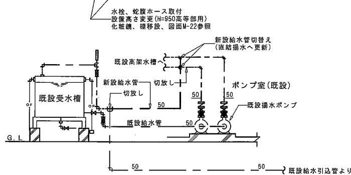
給水引込管切替系統図(直結) NO SCALE 注：1. 受水槽及び排水ポンプを中止し、直結排水へ配管路改修を行う。 1階衛生設備改修図(新・旧校舎) S=1/150
