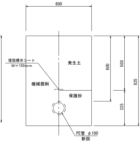
園内土工 ⑪⑦
