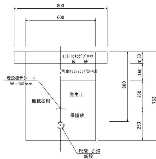
園路土工 ⑩
