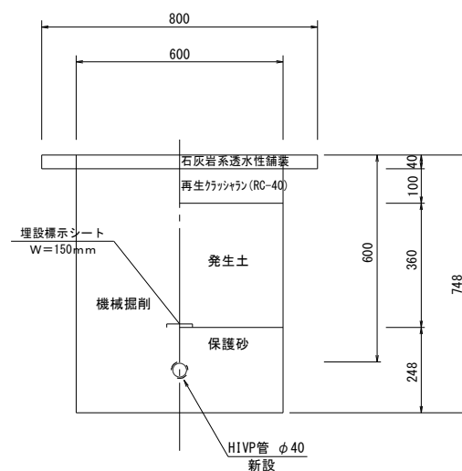
園路土工 ⑭
