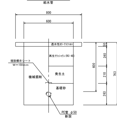
園路土工⑤
