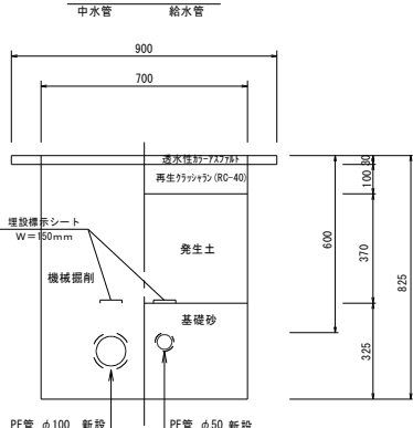
園路土工③
