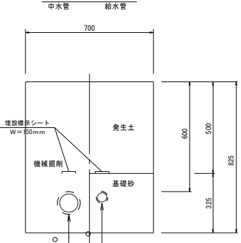
園内土工③
