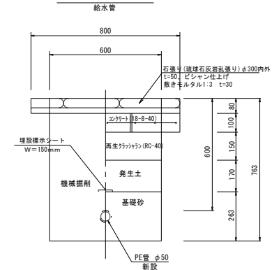
園路土工⑦
