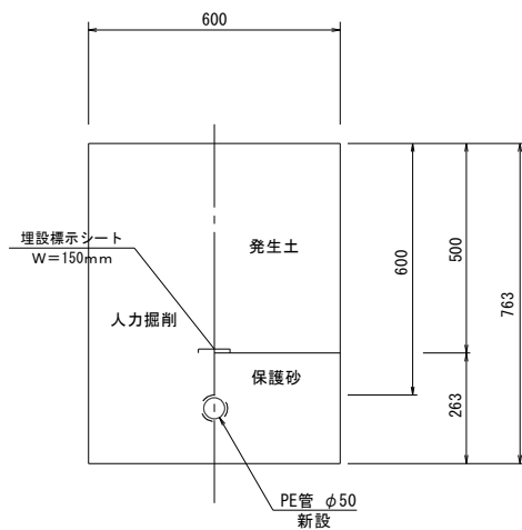
園路土工 ⑪
