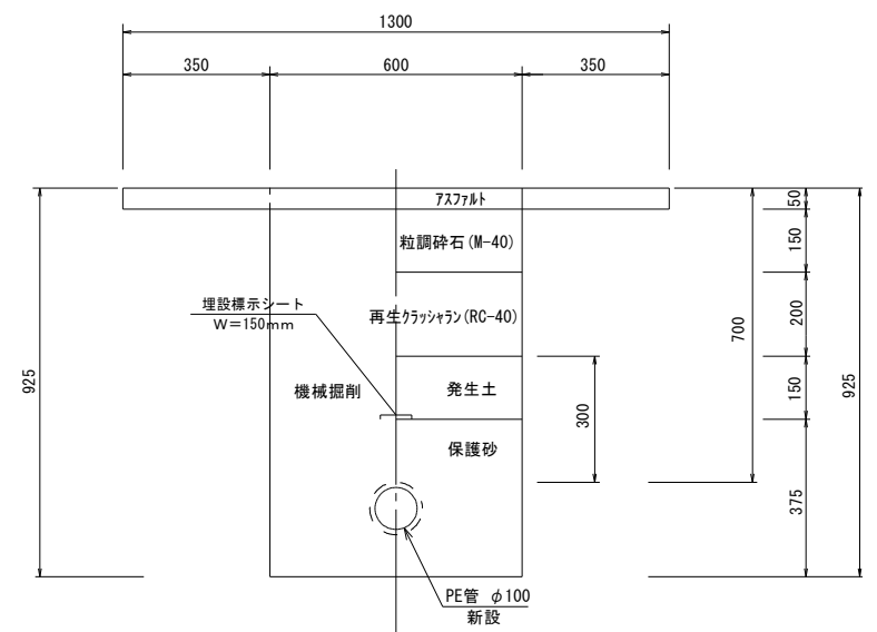
市道土工②
