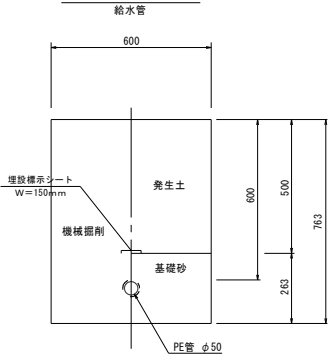
園内土工②
