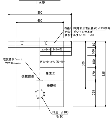
園路土工⑨
