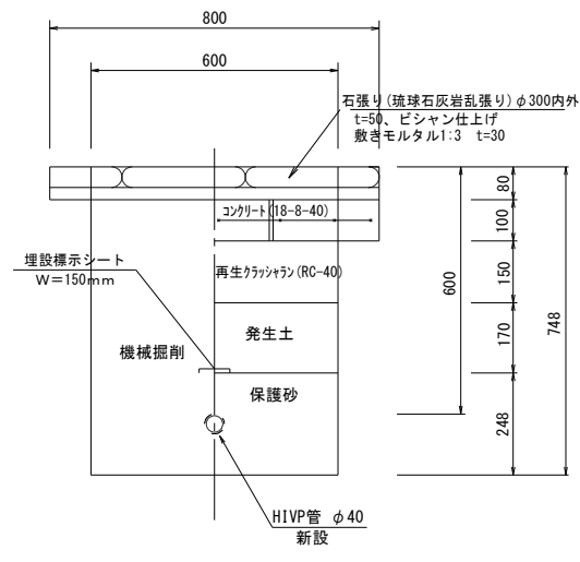
園路土工 ⑭
