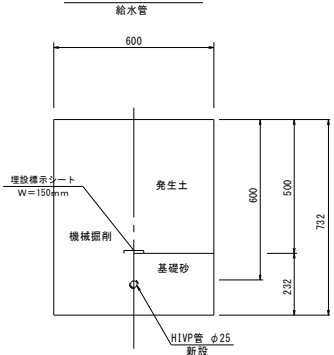
園内土工①
