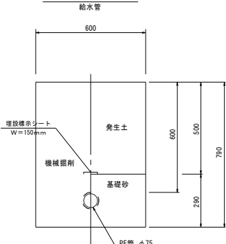
園内土工④
