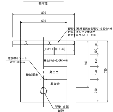
園路土工⑧
