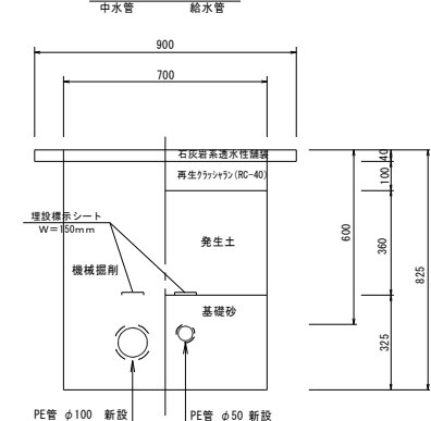
園路土工④
