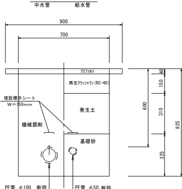
園路土工②
