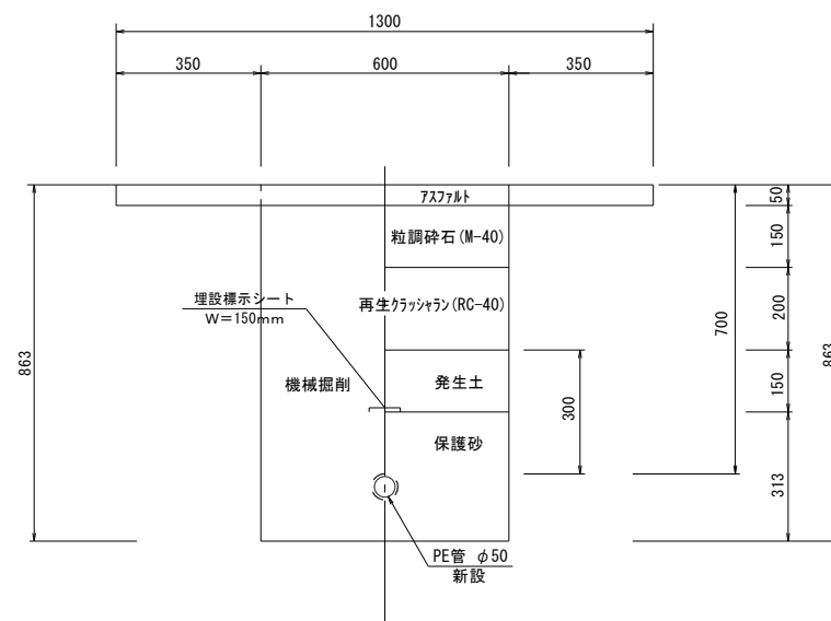
市道土工①
