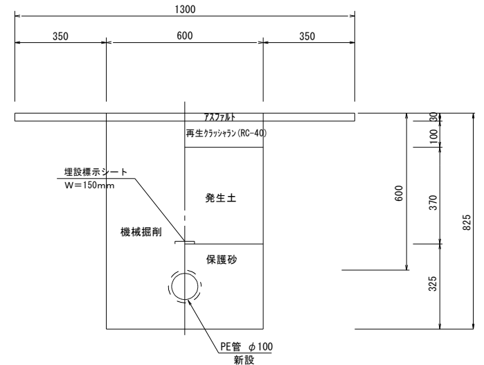
園内土工 ⑪⑦
