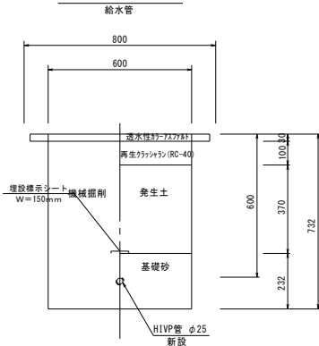
園路土工①
