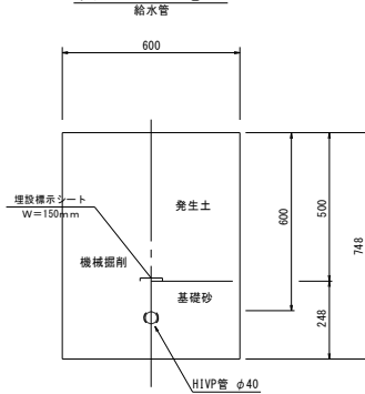
園内土工⑤
