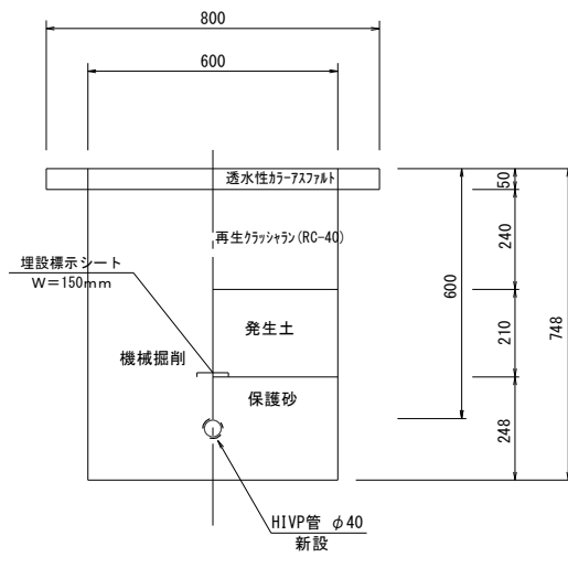
園路土工 ⑬
