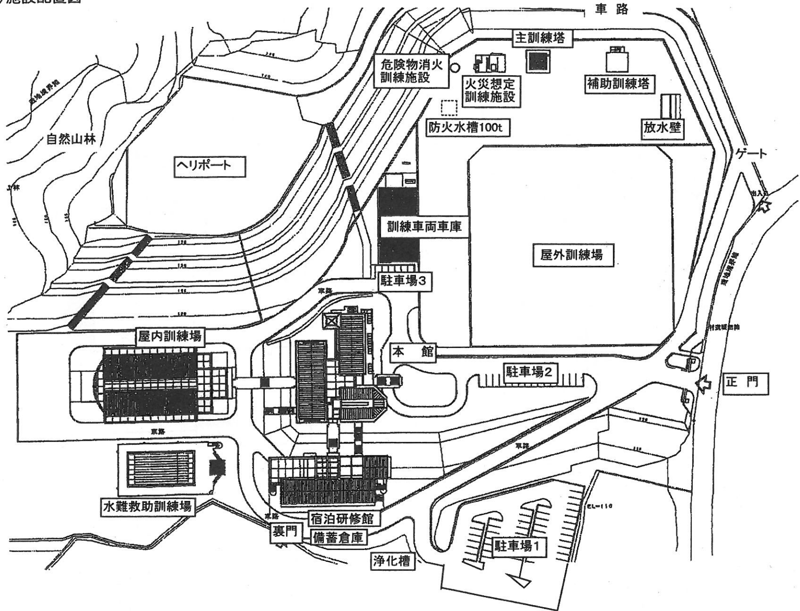
(5)施設配置図
