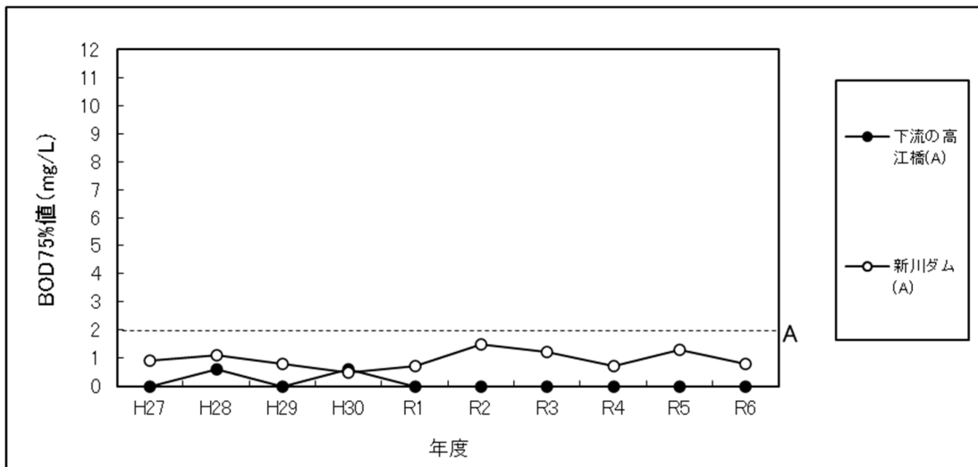
新川川の水質 (BOD75%値) 経年変化
