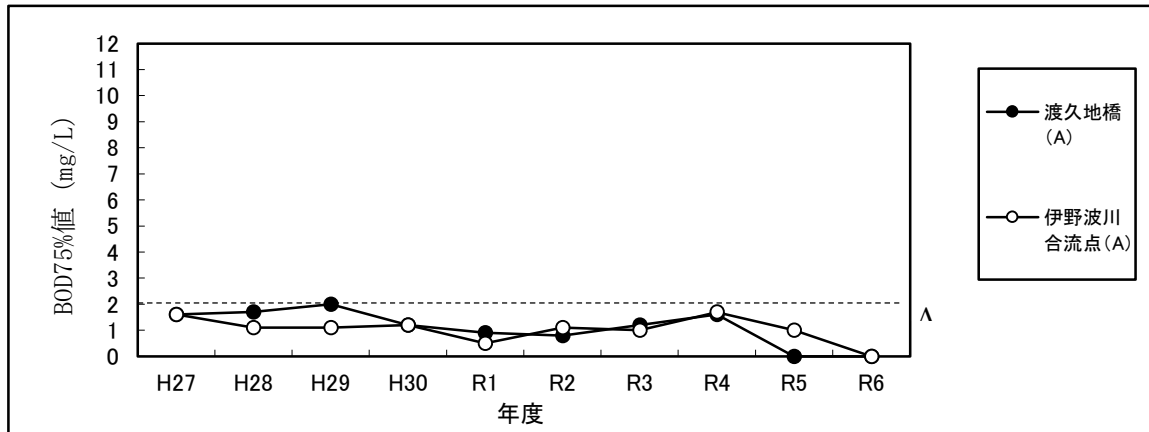
満名川の水質 (BOD75%値) 経年変化
