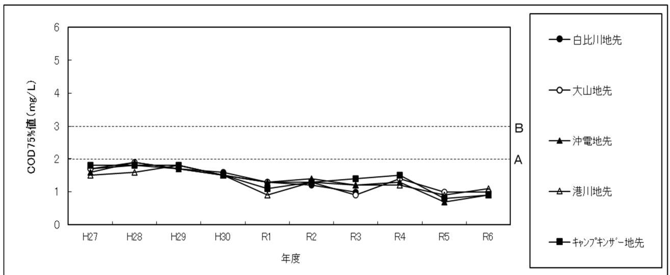
伊佐海域の水質 (COD 値) 経年変化
