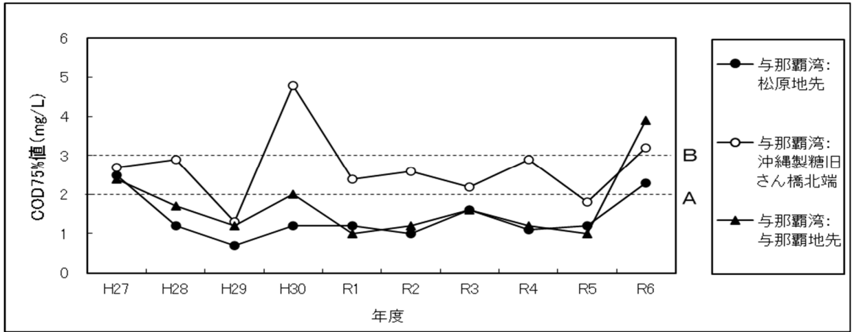
与那覇湾の水質 (COD 値) 経年変化
