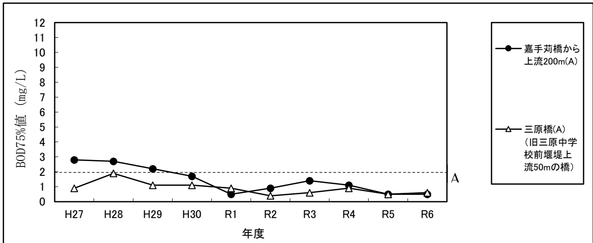
汀間川の水質 (BOD75%値) 経年変化
