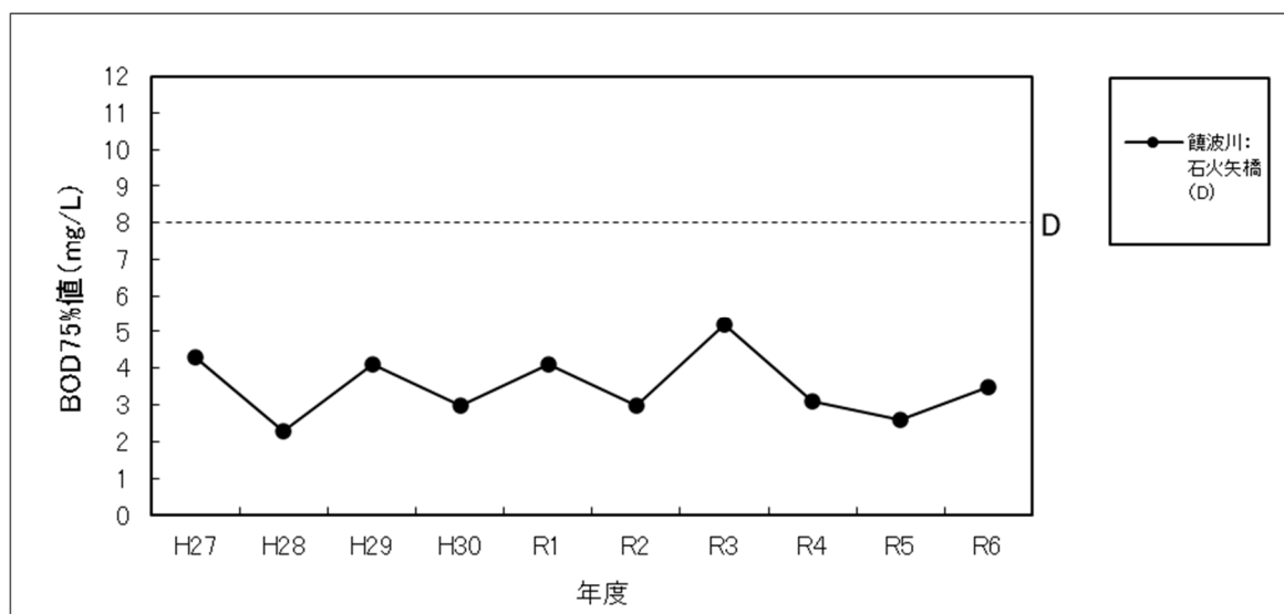
饒波川の水質（BOD75%値）経年変化
