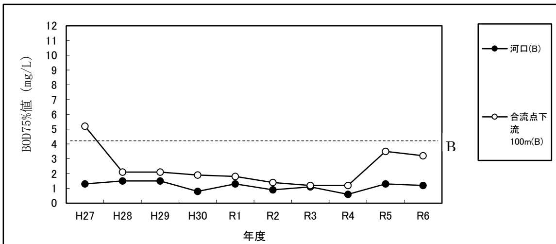
天願川の水質 (BOD75%値) 経年変化
