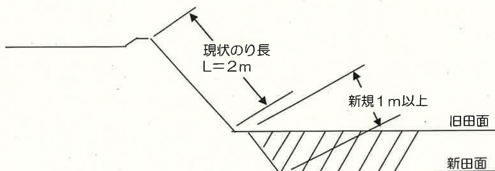
【法 18 条 1 項 3 号に該当するのり切・切土】
