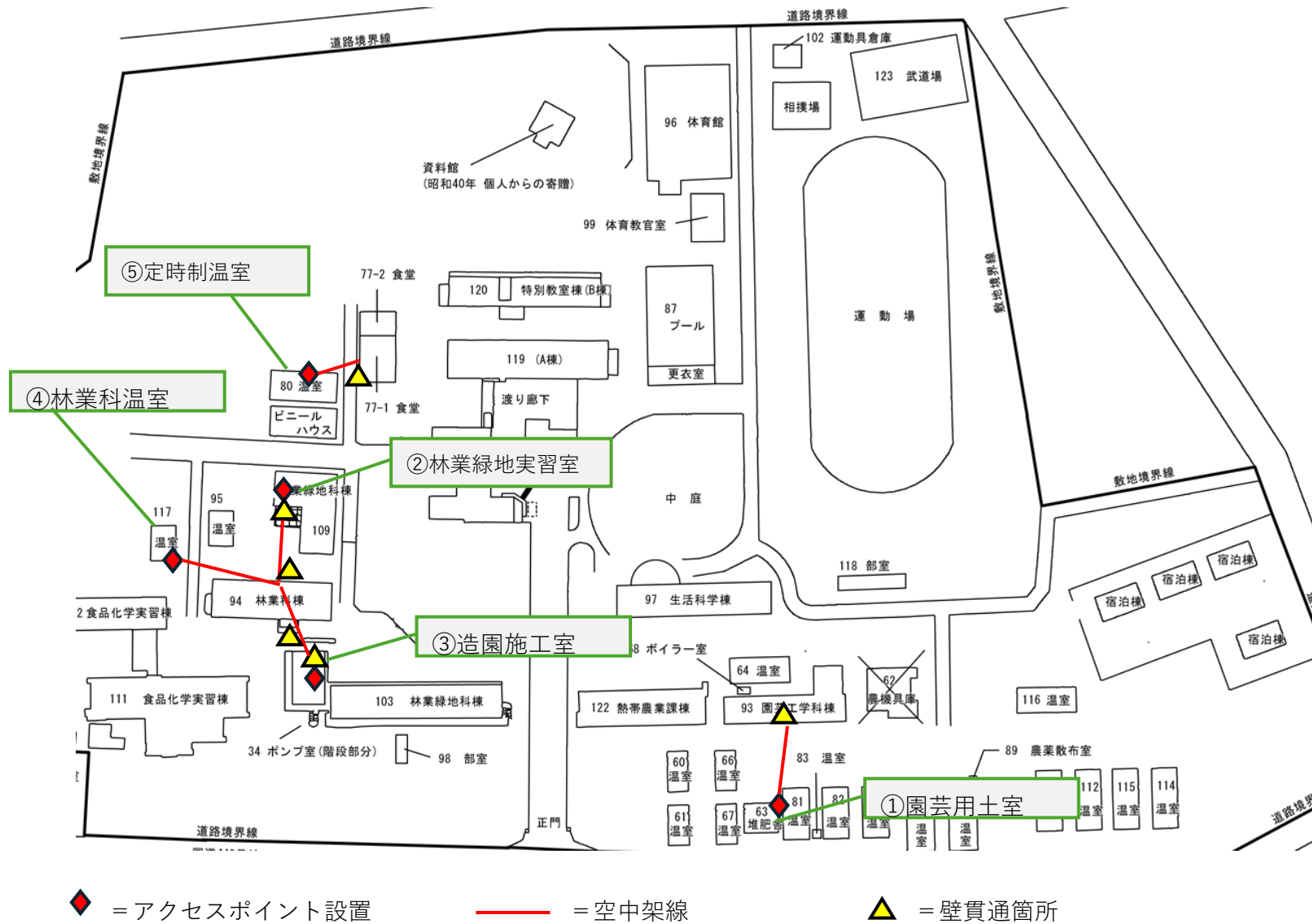
北部農林高校 LAN配線及びアクセスポイント設置図
