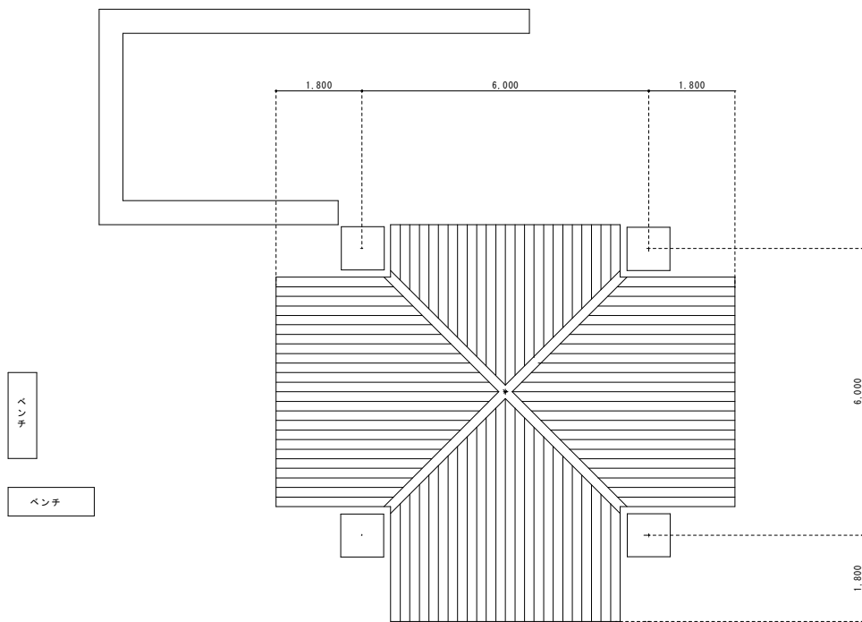
屋根伏図
