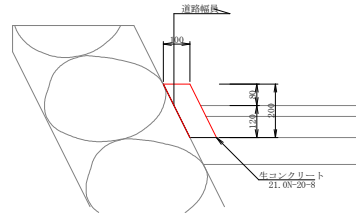
B型舗装止めコンクリート (H=0.12m) S=1/10
