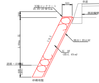
石積工 (H=2.00m迄) ※( )は道路
