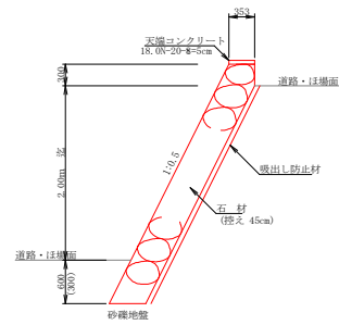
石積工 (H=2.00m迄) ※( )は道路
