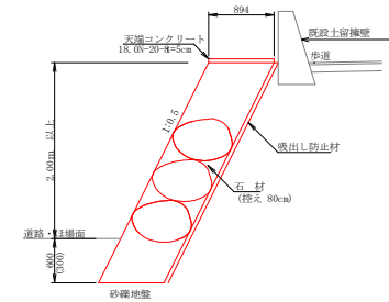
石積工 (H=2.00m以上) ※( )は道路
