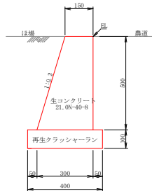
鉋止工 (H=0.50m) S=1/10
