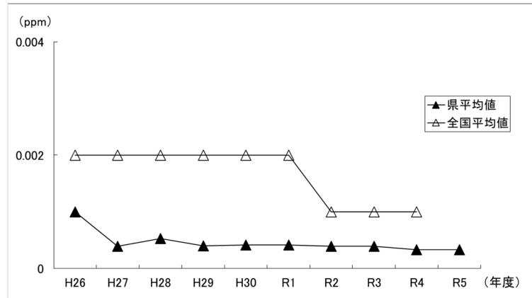
図 1-1-2 二酸化硫黄濃度の経年変化
