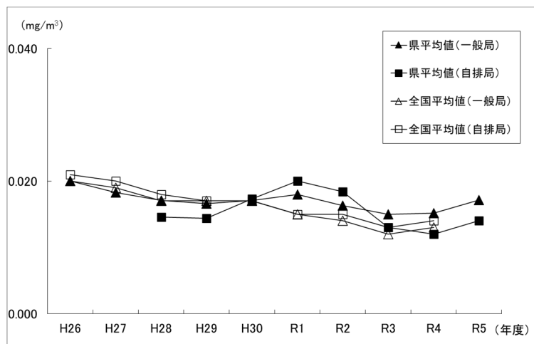
図1-1-4 浮遊粒子状物質濃度の経年変化
