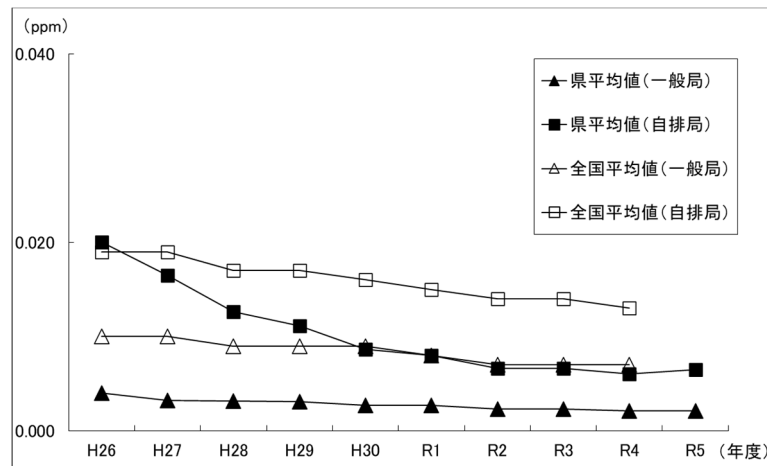
図 1-1-3 二酸化窒素濃度の経年変化
