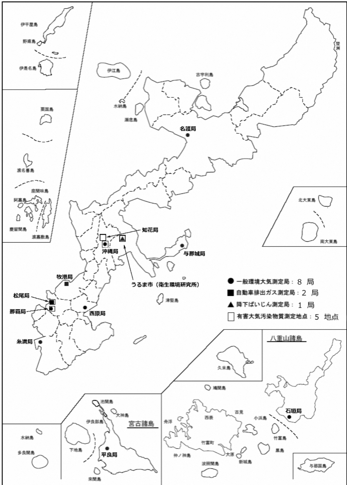
図1-1-1 令和5年度大気汚染常時監視測定局配置図
