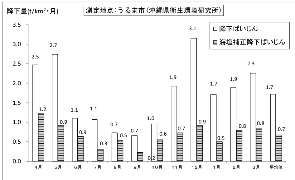
図1-1-9 令和5年度降下ばいじん測定結果
