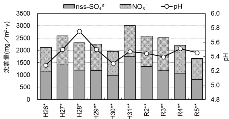
図1-1-11 pH及び \text{nss-SO}_4^{2-} 、 \text{NO}_3^- 沈着量（平成26年度～令和5年度）
