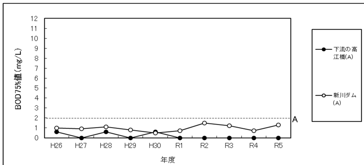
新川川の水質 (BOD75%値) 経年変化
