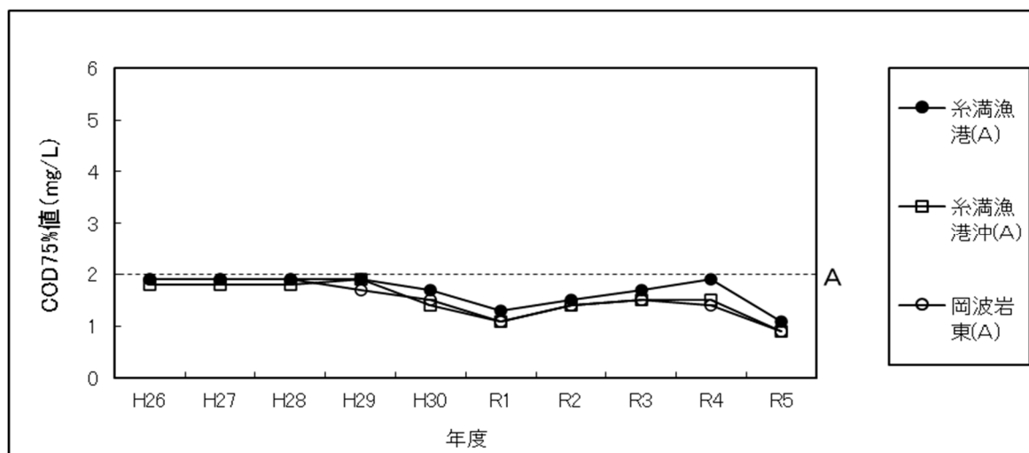
糸満海域の水質 (COD75%値) 経年変化
