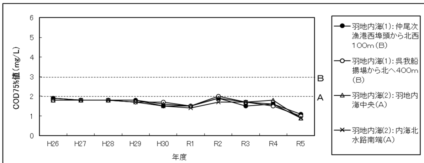
羽地内海(1)及び(2)の水質 (COD75%値) 経年変化
