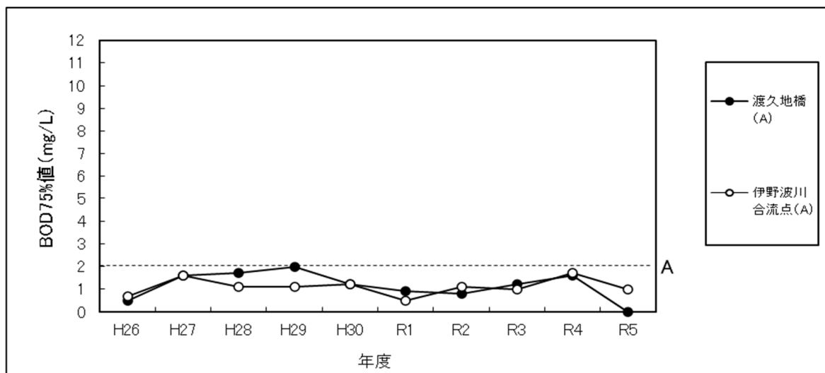
満名川の水質（BOD75%値）経年変化
