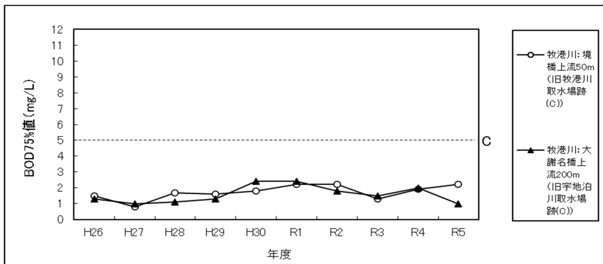
牧港川の水質 (BOD75%値) 経年変化
