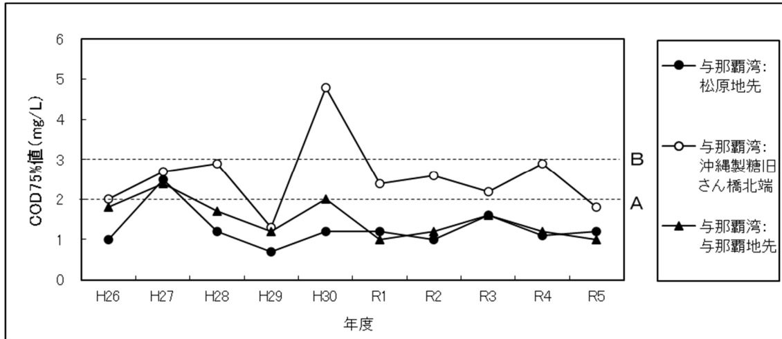
与那覇湾の水質 (COD 値) 経年変化
