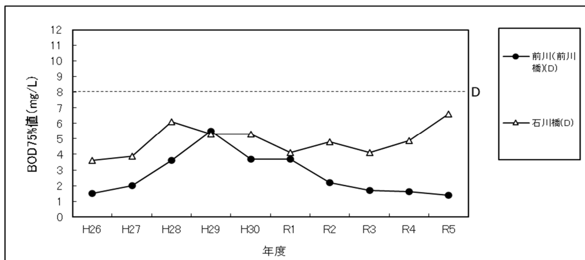
雄樋川の水質（BOD75%値）経年変化
