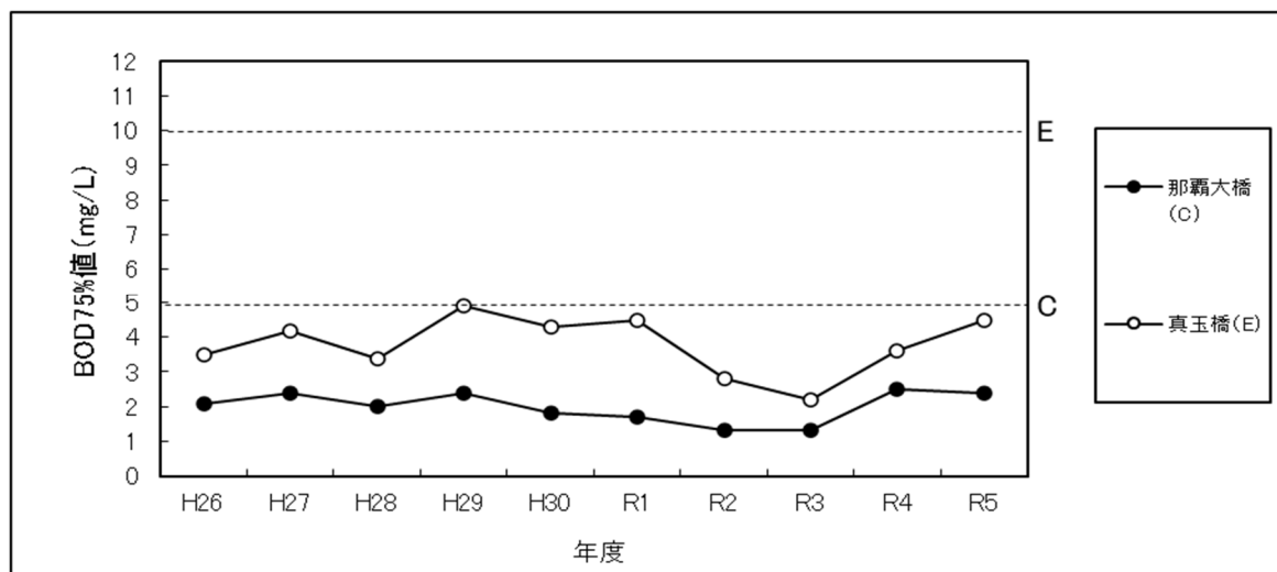
国場川の水質（BOD75%値）経年変化
