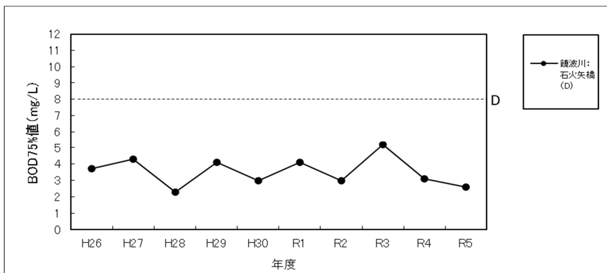
饒波川の水質 (BOD75%値) 経年変化
