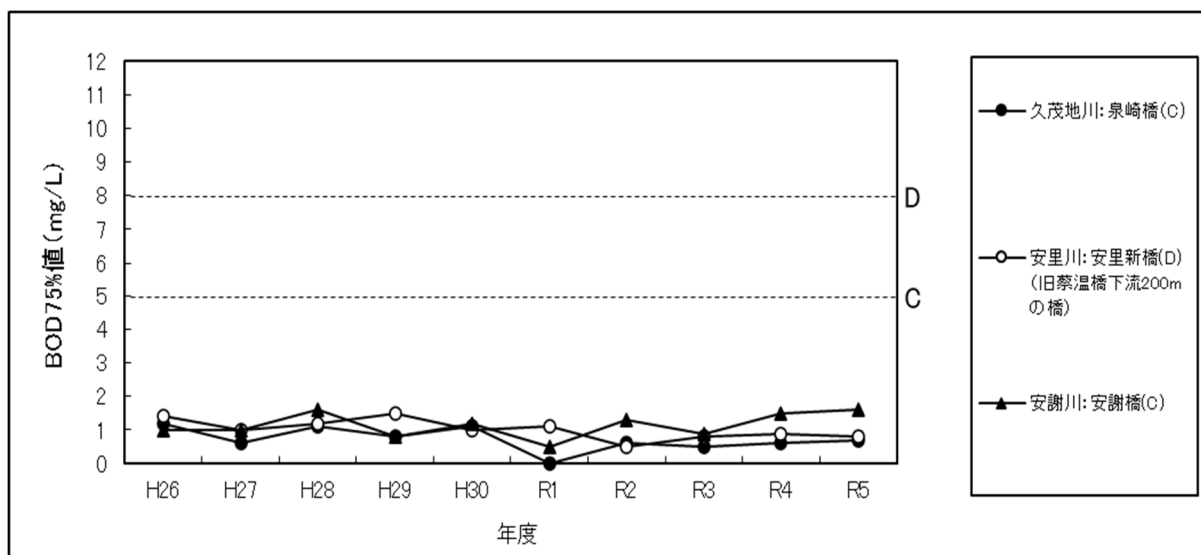
久茂地川・安里川・安謝川の水質 (BOD75%値) 経年変化
