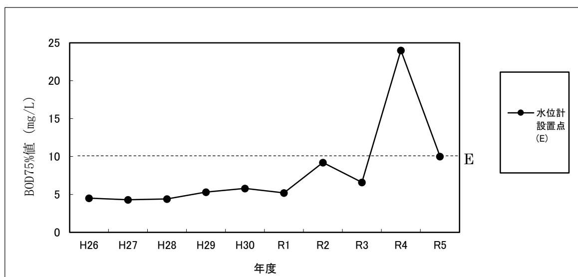
報得川の水質 (BOD75%値) 経年変化
