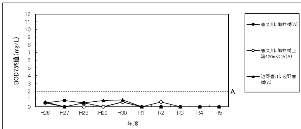
普久川、辺野喜川の水質 (BOD75%値) 経年変化
