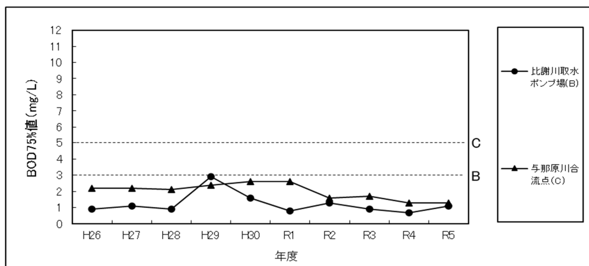
比謝川の水質（BOD75%値）経年変化
