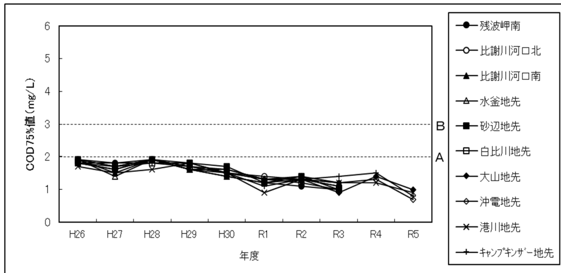
伊佐海域の水質 (COD 値) 経年変化
