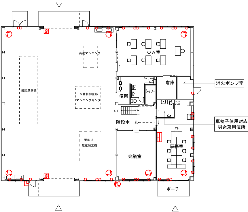
1 階
