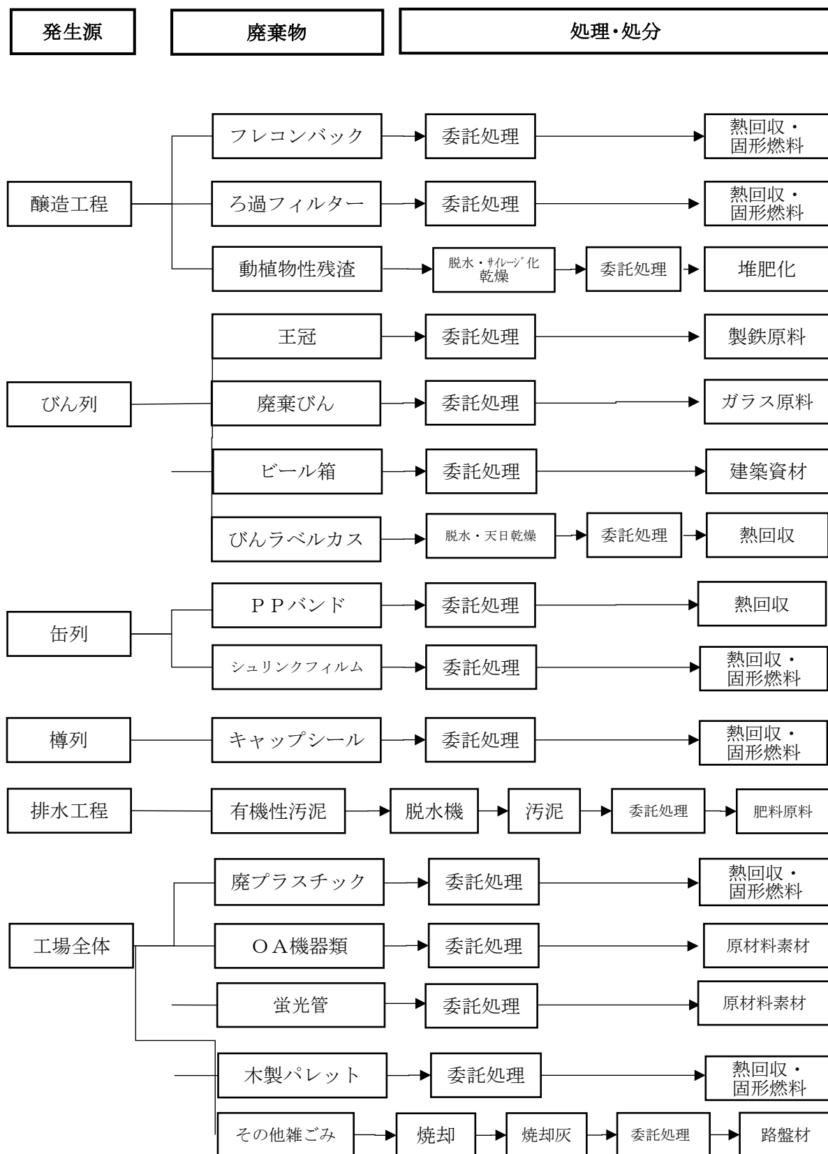
別表1 廃棄物処理フローシート
