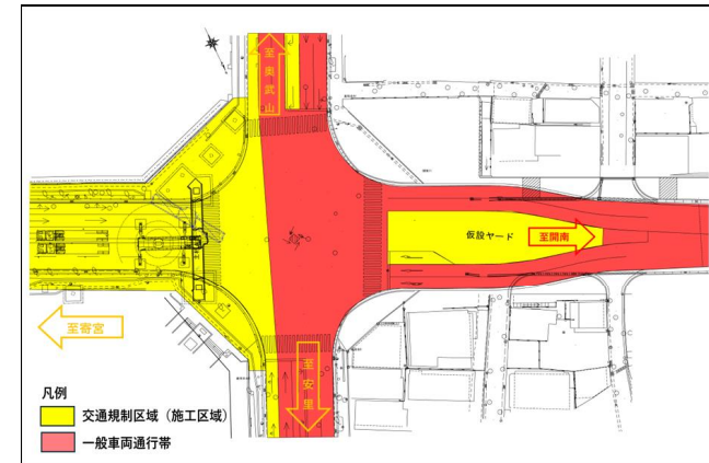
迂回路ルート
