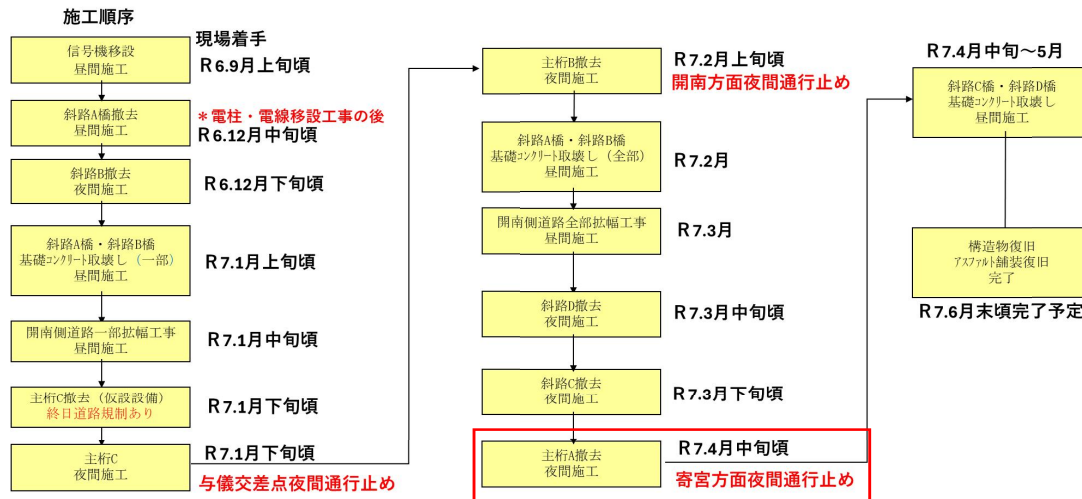
主桁A撤去 (夜間施工)
