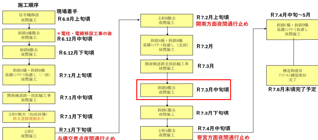
寄宮川歩道迂回路設置 (R7.2月～R7.5月頃)
