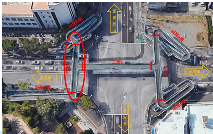
主桁A撤去 (夜間施工)
