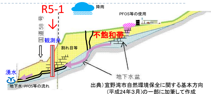
下流側湧水～飛行場の断面図
