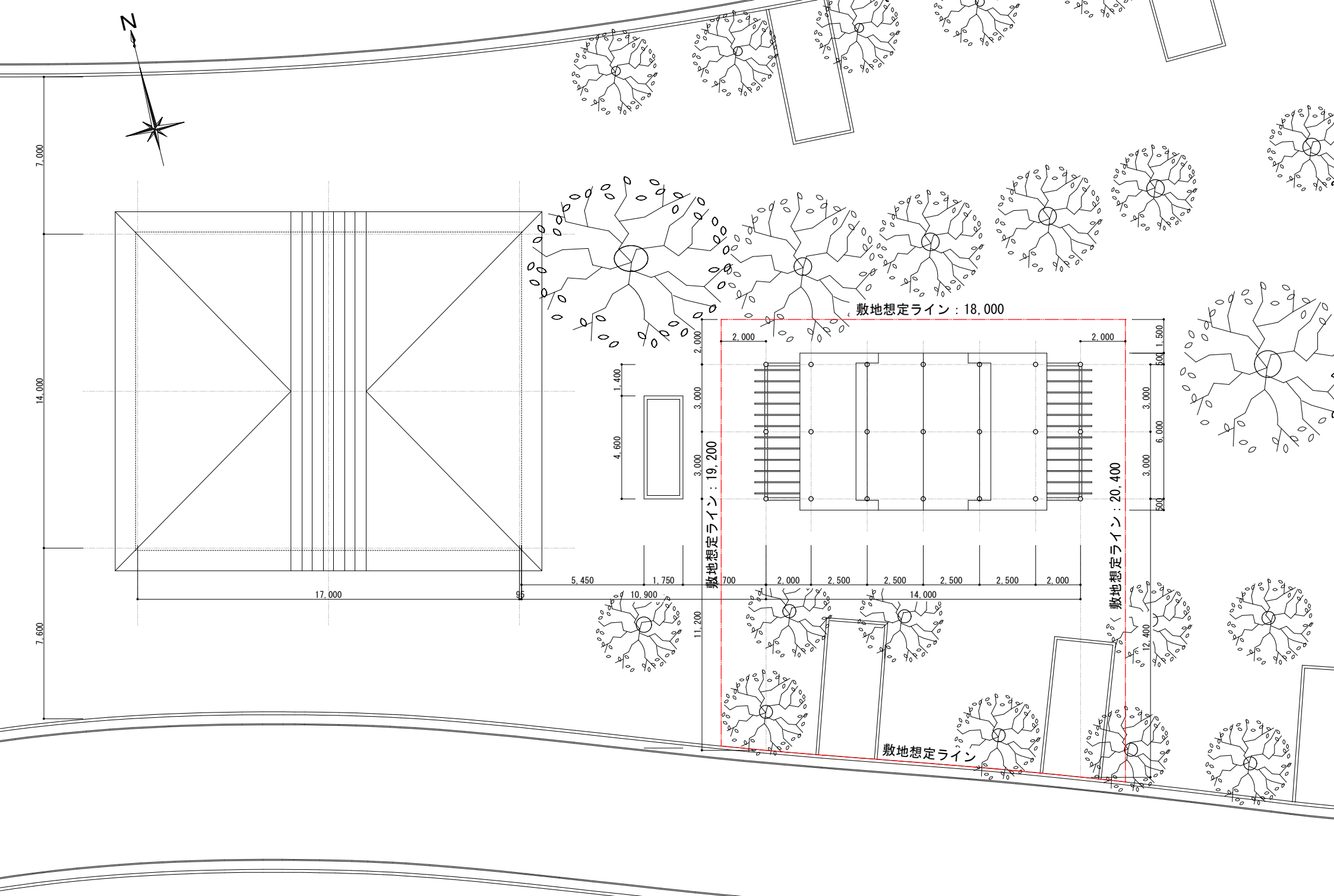
現況配置図 S=1/200
