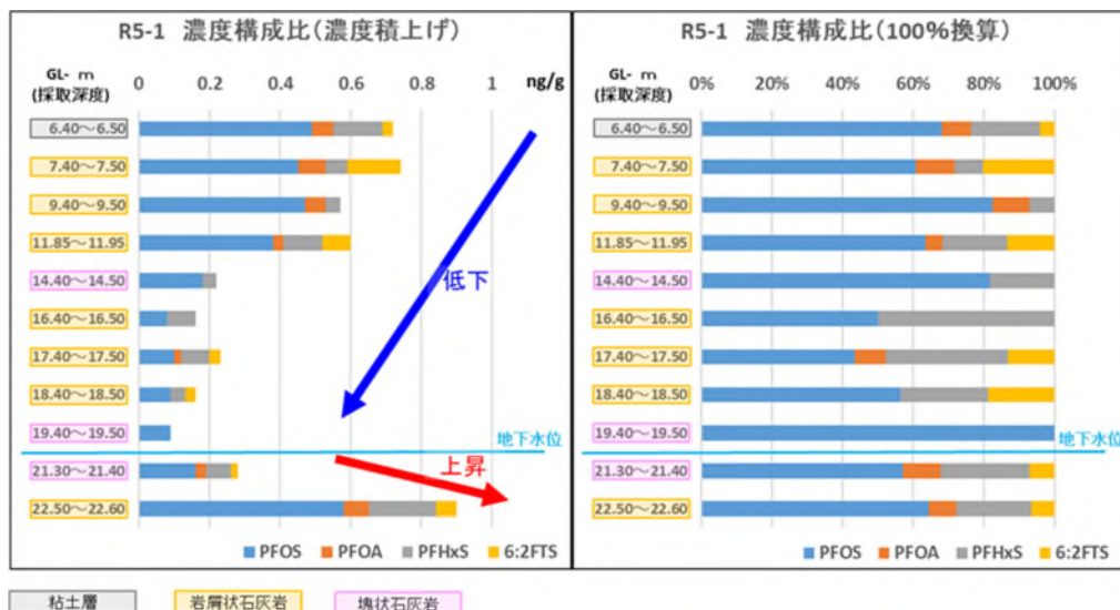
図 2.5.5 深度方向の石灰岩等における PFOS 等の濃度構成比（R5-1 孔）
