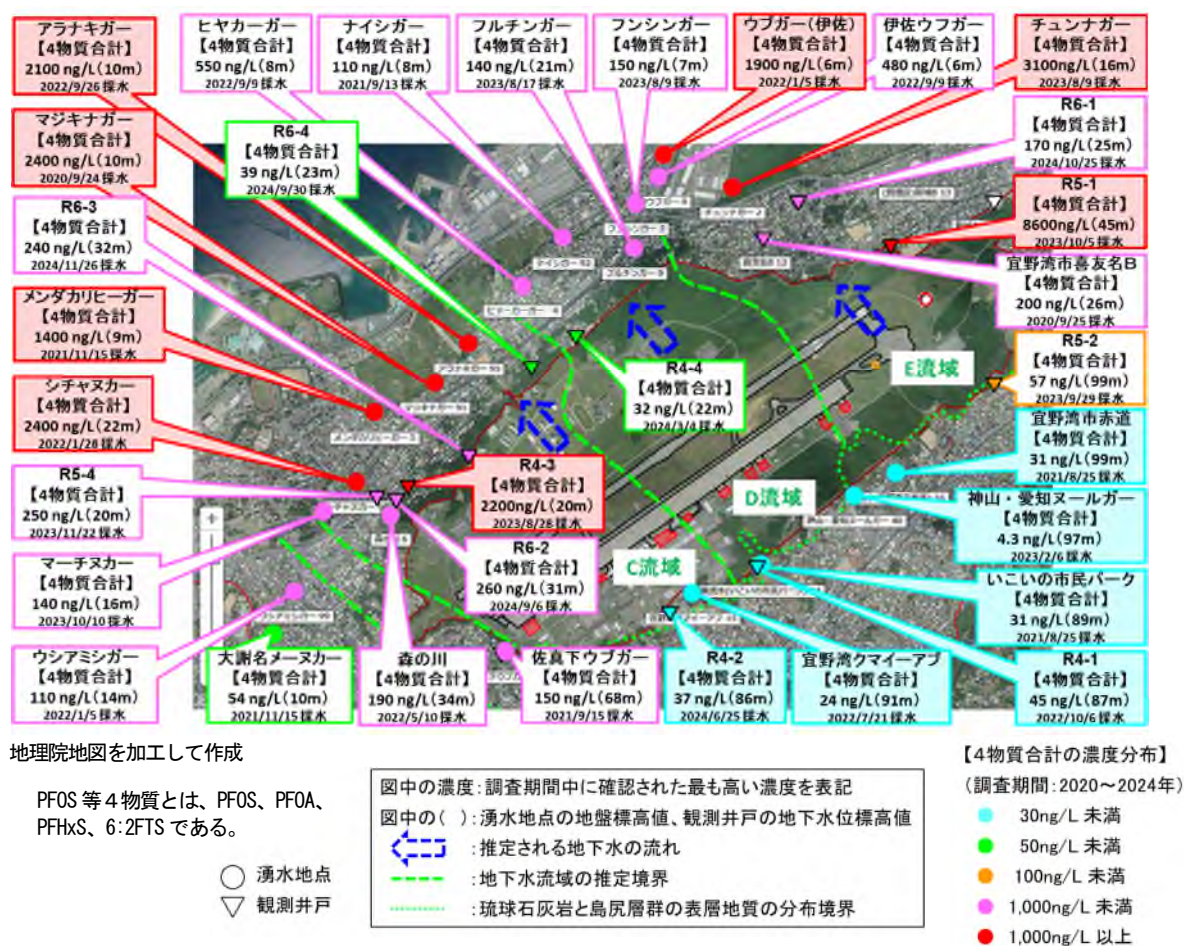
図 2.4.1 地下水流域界と PFOS 等 (4 物質の合計値) の濃度分布
