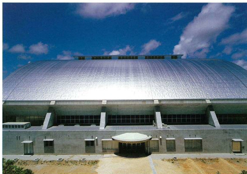
東面外観
