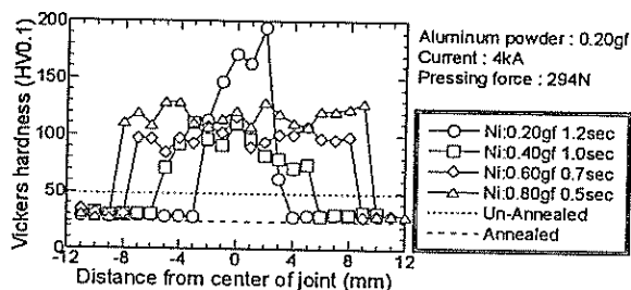
図7 硬さ試験結果
