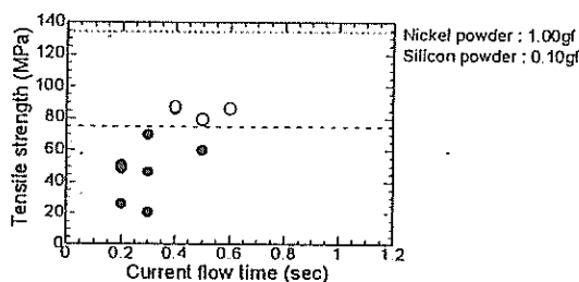
図9 引張試験結果
