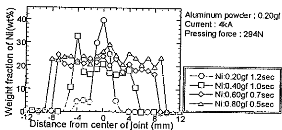
図8 定量分析結果
