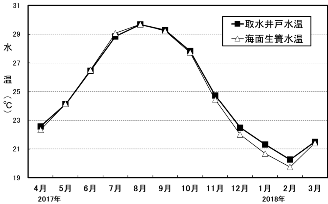
資料6 平成 29(2017)年度の取水井戸及び海面生簀の月平均水温の推移
