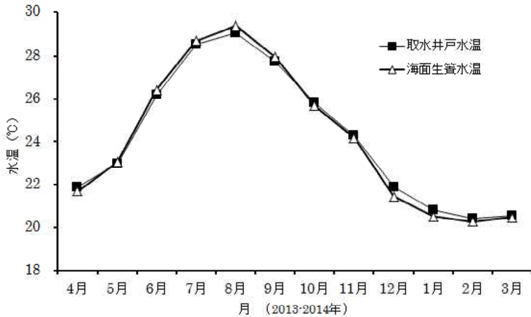
資料6 栽培漁業センター取水井戸及び海面生簀の月平均水温の推移
