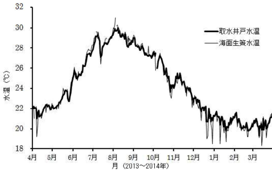
資料7 栽培漁業センター取水井戸及び海面生簀の日水温の推移
