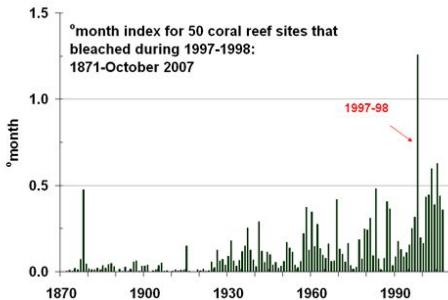
図4-2-3. 世界のサンゴ礁 50 ヶ所における高水温指数(UK Hadley Centre global monthly SST;1871-1999とNOAA NCEP EMC CMB Global Reyn-Smith Olv2 Satellite and observations data setをもとに作成). °monthは1982年から1999年のデータをもとに、年間の月々の平均最大水温を超える月を合計した高水温指数. 解析の詳細はLough(2000)を参照. オーストラリア海洋科学研究所ホームページより.
