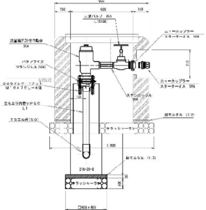
農業用排水施設（給水栓）
