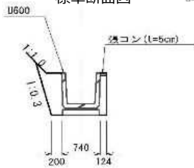
標準断面図
