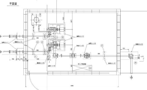
揚水機場
