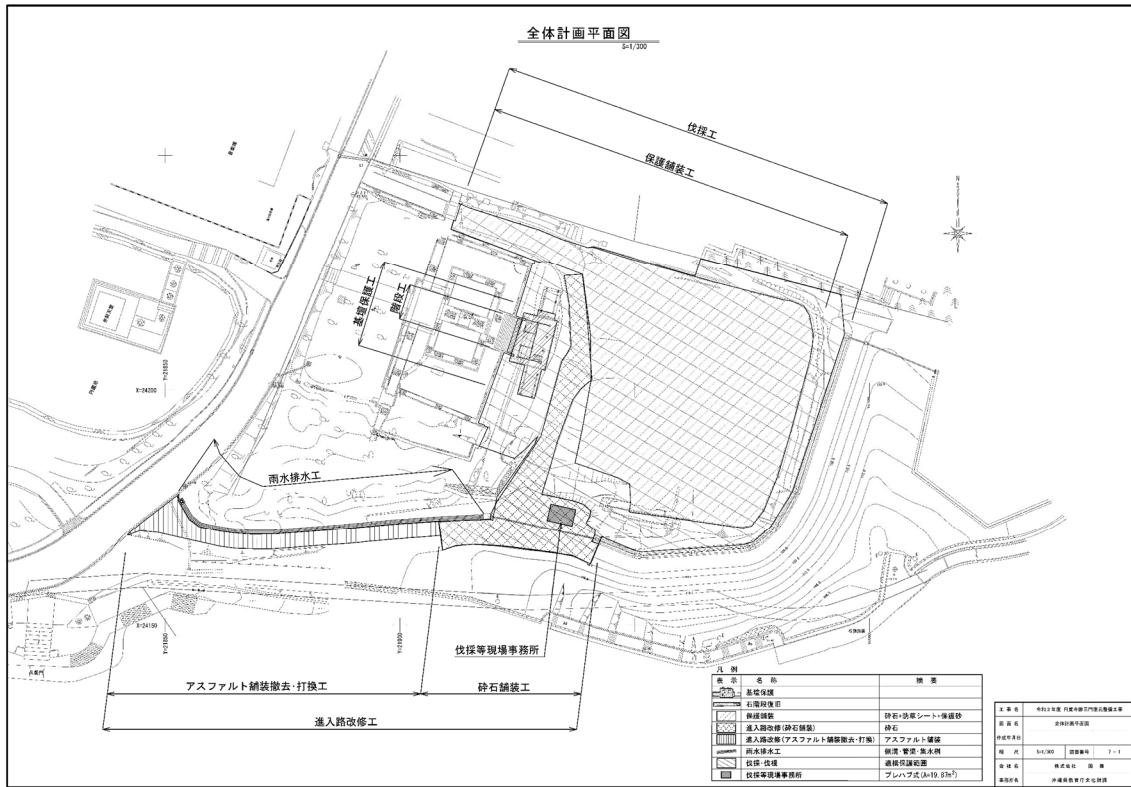
円覚寺跡三門復元整備工事 全体計画平面図
