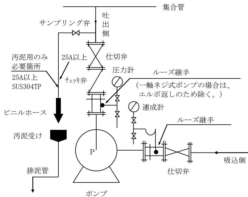
ポンプ周り参考図
