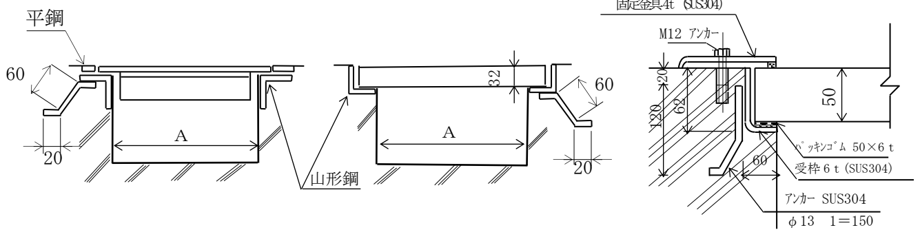
縞鋼板蓋参考図
