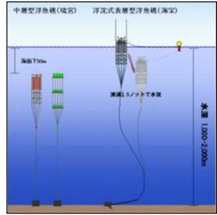
浮沈式表層型浮魚礁
