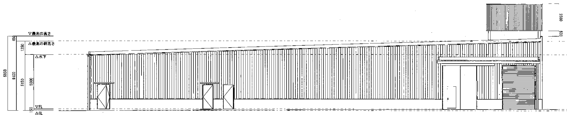
北東側立面図
