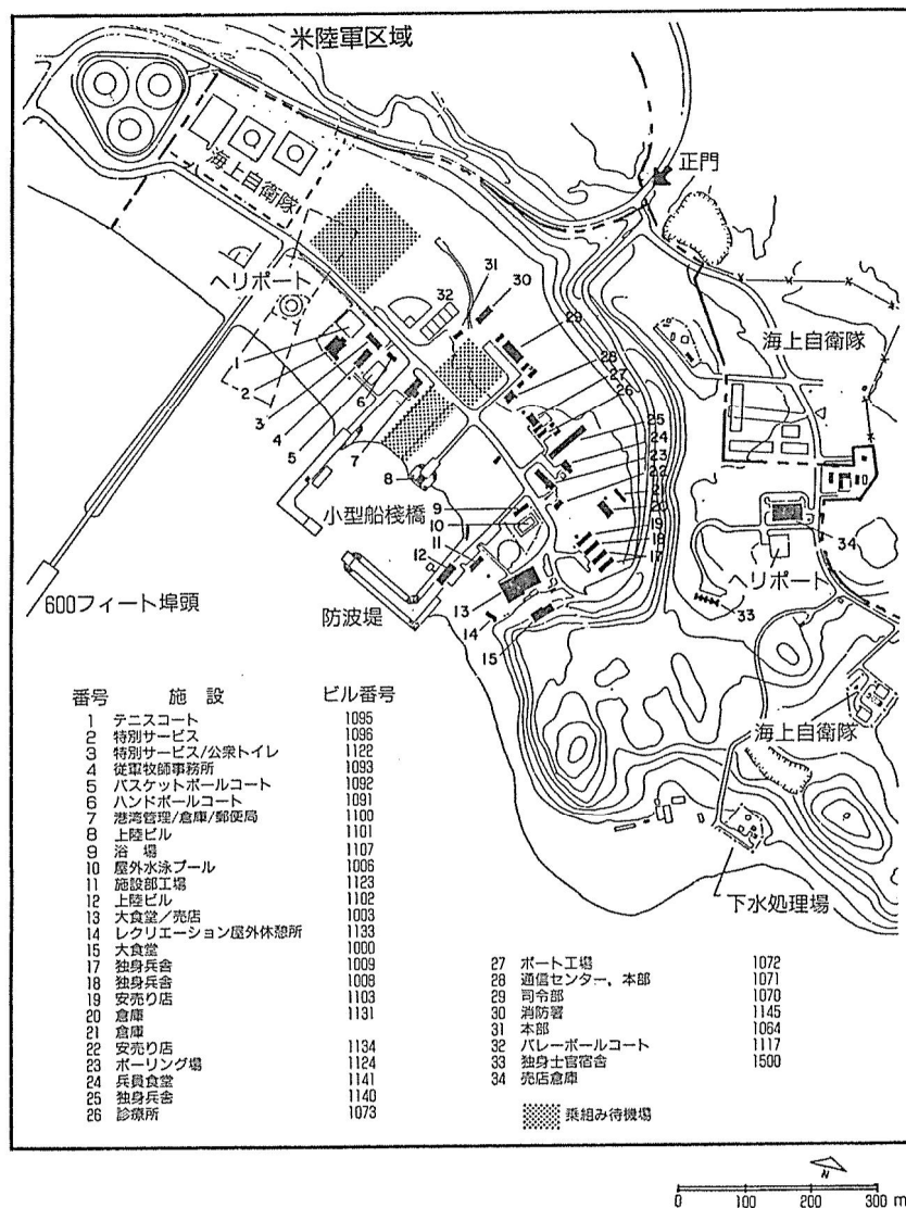
図46-4 ホワイト・ビーチ地区の施設配置図
