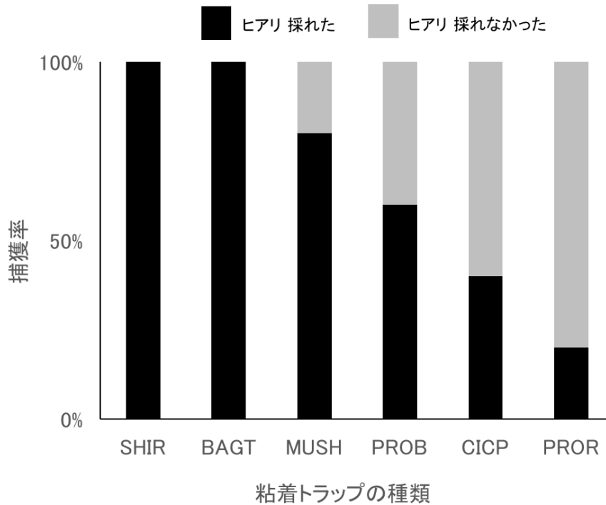
図 1-3_6 各種粘着トラップのヒアリ捕獲率
