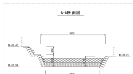
図-2.4.16 フトン籠の設置工程④(恩納村試験地)
