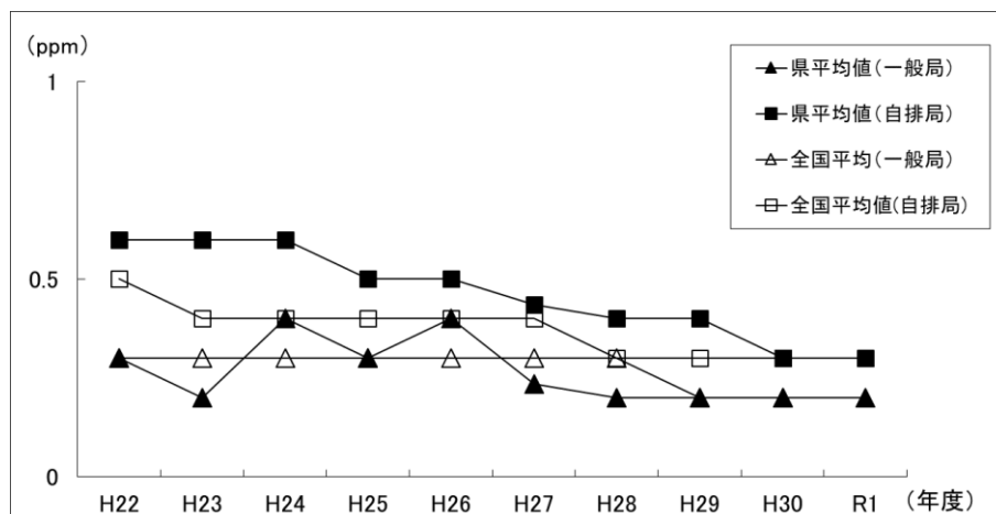
図 1-1-5 一酸化炭素濃度の経年変化
