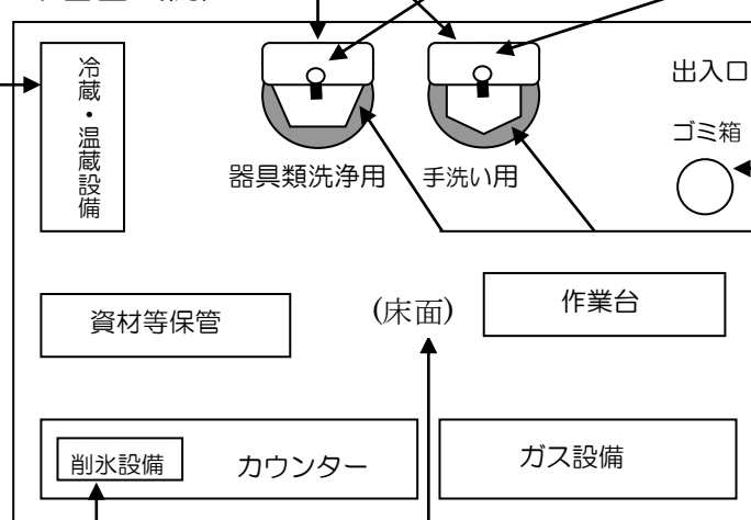
平面図（例）
