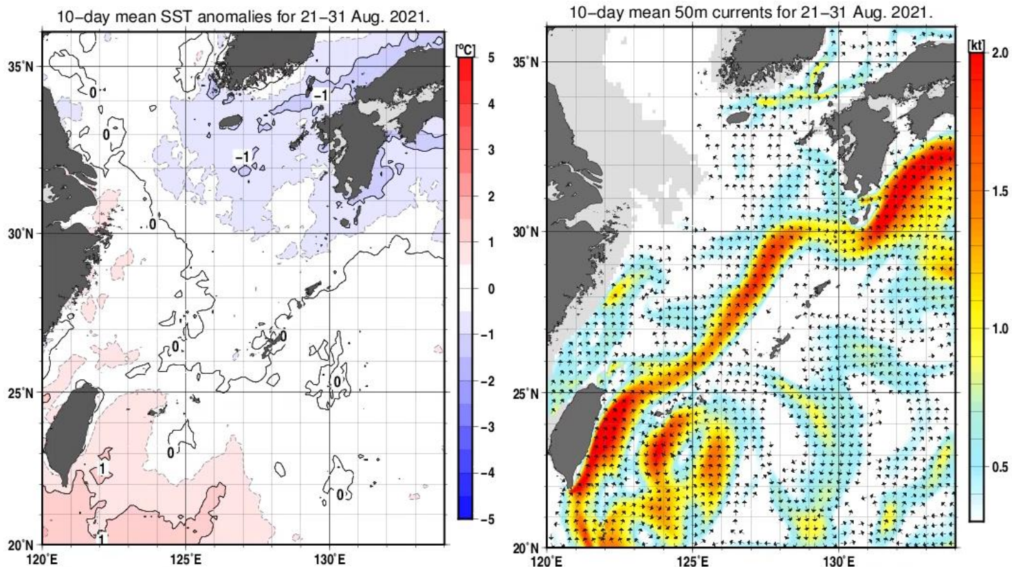
図2. 2021年8月下旬海面水温偏差図(左)及び海流図(気象庁HPより)
