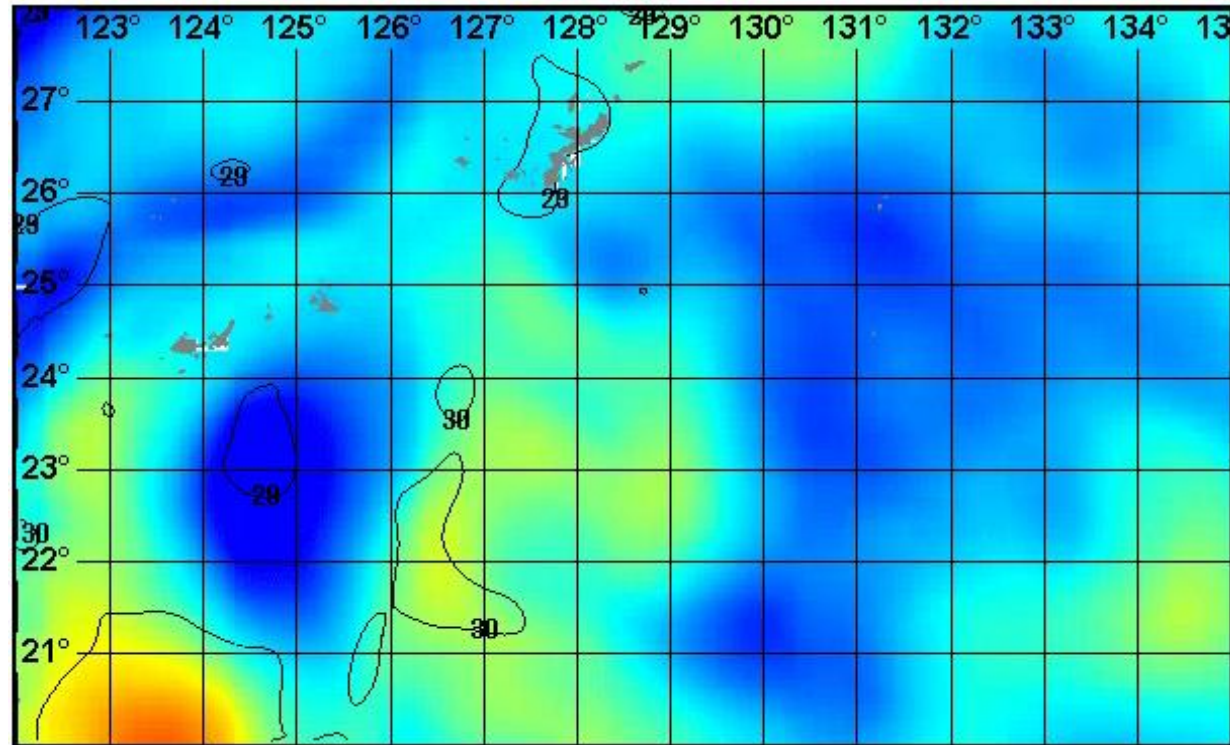
図1. 海況案内人による表面水温(等温度線)・海面高度分布(塗り分け)図(2021年8月31日)
