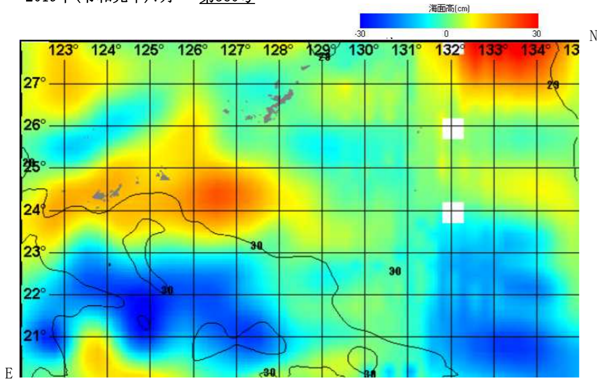
図1. 海況案内人による表面水温(等温度線)・海面高度分布(塗り分け)図(2019年7月31日)
