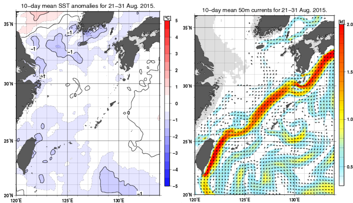
図2. 2015年8月下旬海面水温偏差図(左)及び海流図(気象庁HPより)
