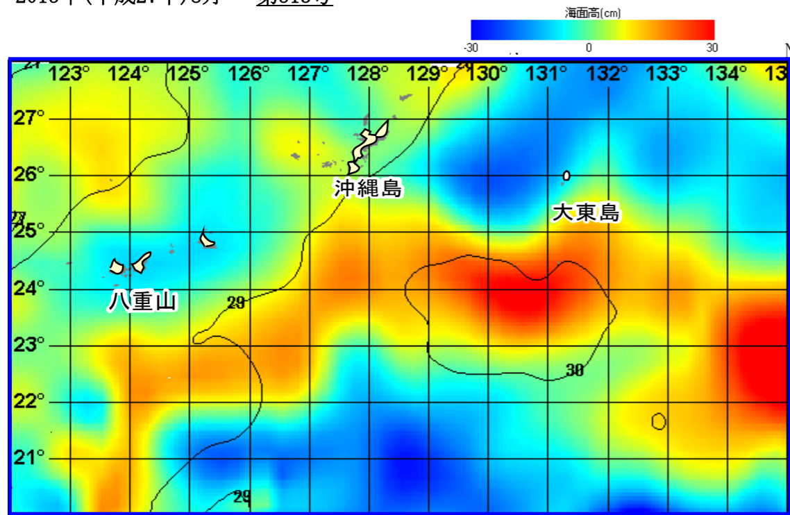
図1. 海況案内人による表面水温(等温度線)・海面高度分布(塗り分け)図(2015年8月31日)
