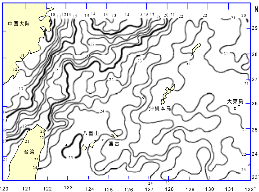
図1 表面水温分布図(2004年3月16日)
