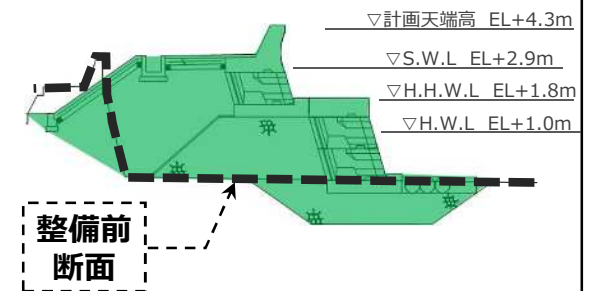
標準断面図 (一般部)
