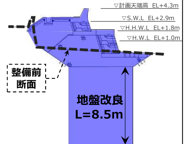
標準断面図 (地盤改良部)
