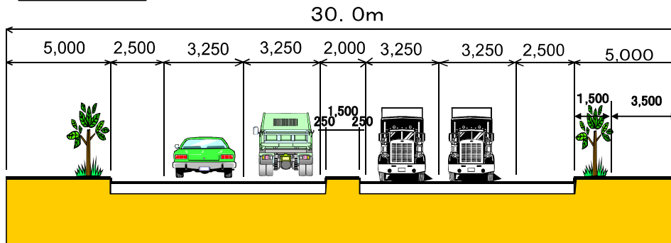
計画幅員
