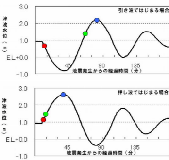
図2 津波影響開始時間、到達時間説明図
