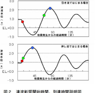
図2 津波影響開始時間、到達時間説明図
