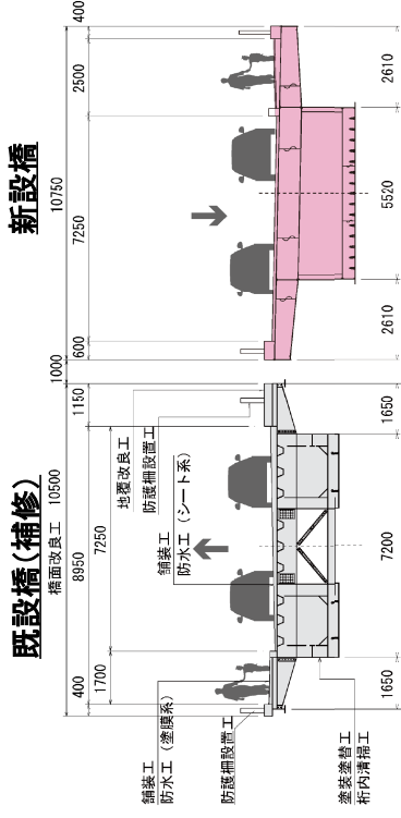
上部工断面図
