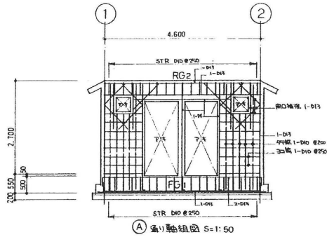
① A 通り軸組図 S=1:50
