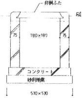
弁掛 (VC-1)
