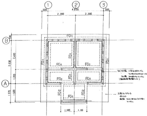
基礎伏図 S=1:50
