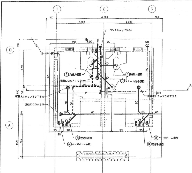
便所内設備平面図 S=1:30
