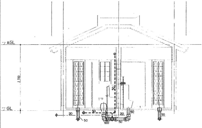
A~A断面図 S=1:30
