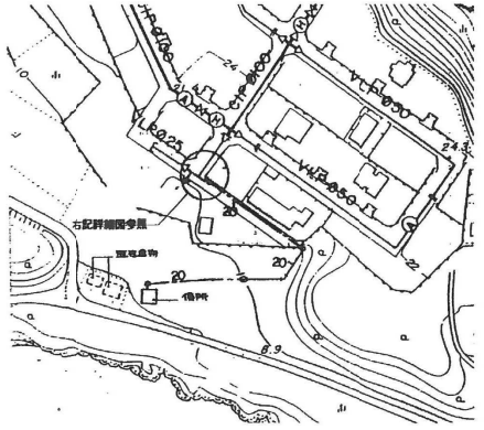
給水管引込詳細図 NOSCALE
