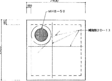
溜掛平面図 S=1:30
