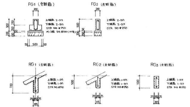
部材リスト S=1:30
