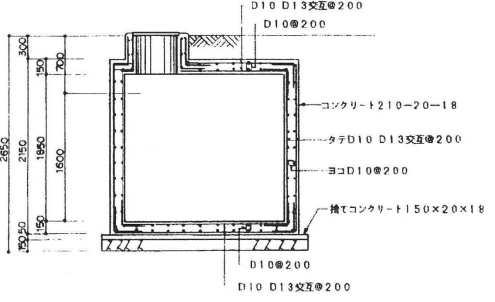
溜掛断面図 S=1:30
