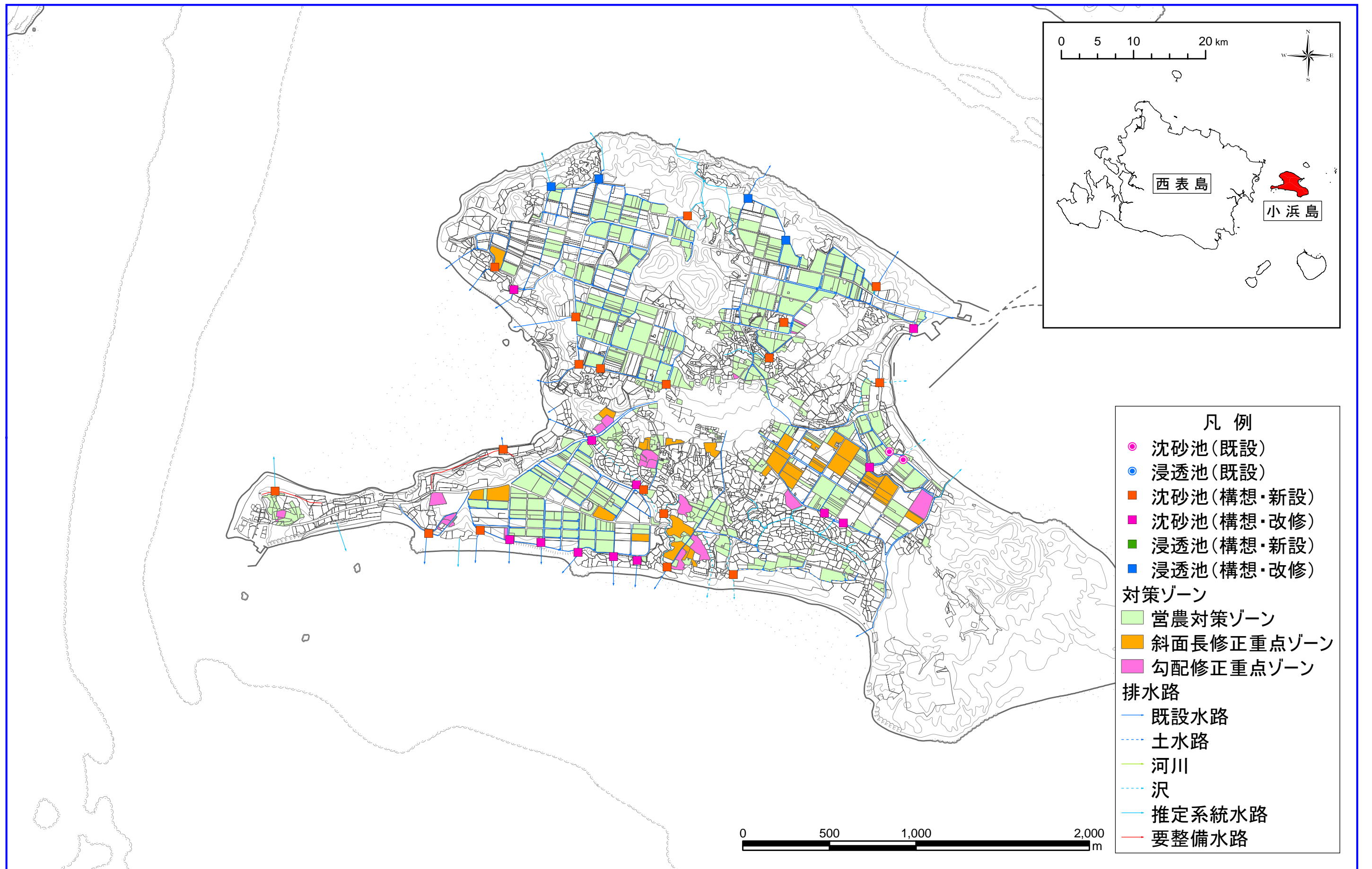
図2-22 竹富町小浜島要整備構想図
