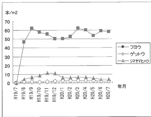
図-1 生立本数（切土法面）
