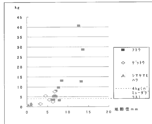
図-4 引抜強度（盛土法面）
