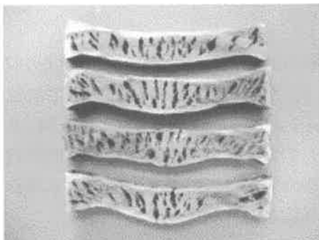
写真-1 断面変形及び内部割れ
