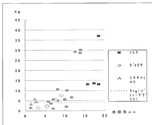
図-3 引抜強度（切土法面）
