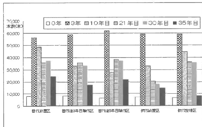
図－2 試験区の立木本数の推移 (全立木)
