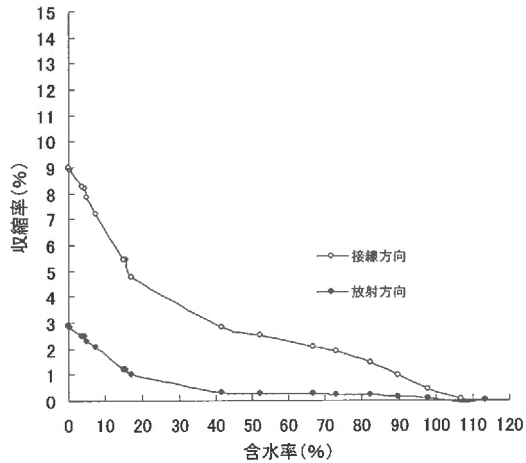
図-1 収縮経過
